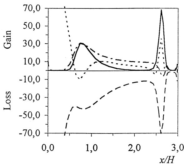
Original \omega -equation.
