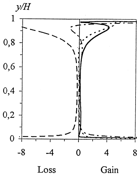
Original \omega -equation.
